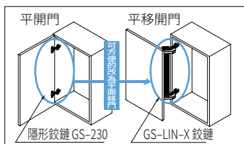
對於使用快裝隱形鉸鏈 GS-230，可直接在門上方便的更換為 GS-LIN-X 鉸鏈
